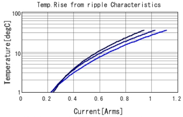
GRM1555C1H270JA01 Temp. rise — 500MHz — 700I
