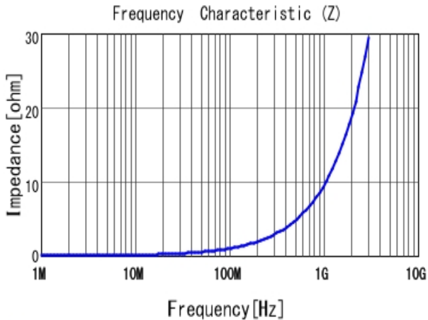
■ LQW15AN1N5C80 |Z|
