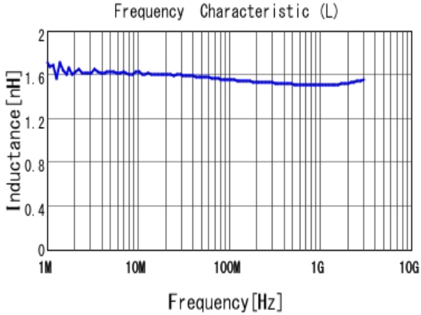
■ LQW15AN1N5C80 L
