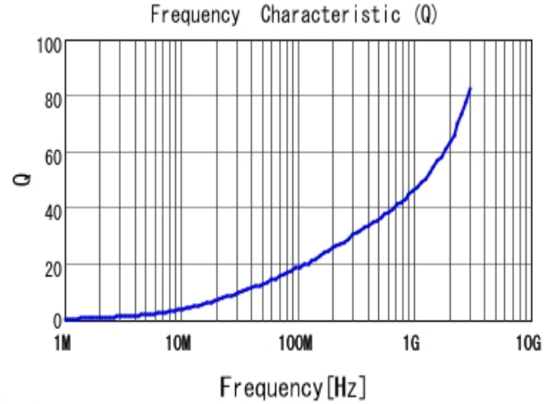
■ LQW15AN1N5C80 Q
