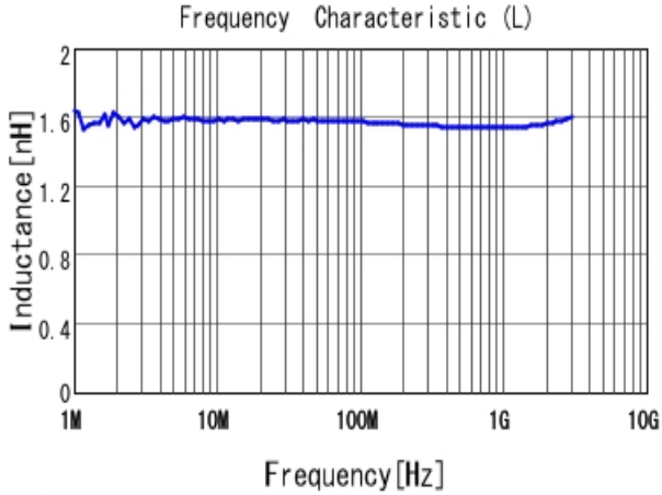
■ LQW15AN1N6C80 L
