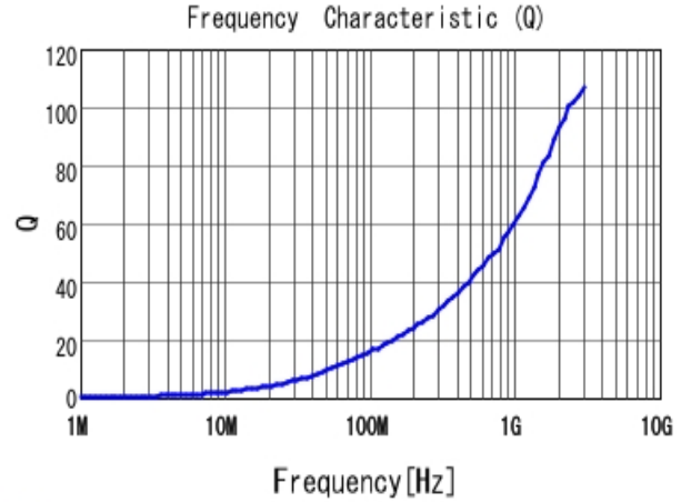
■ LQW15AN1N6D80 Q
