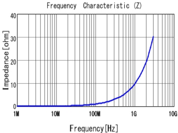
■ LQW15AN1N6D80 |Z|
