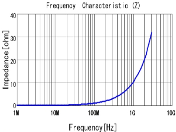
■ LQW15AN1N7D80 |Z|
