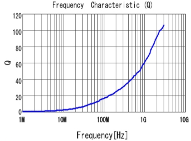
■ LQW15AN1N7D80 Q
