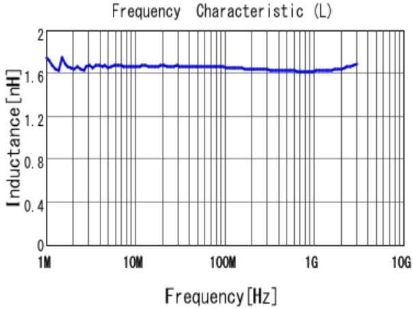
■ LQW15AN1N7D80 L
