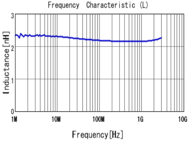
■ LQW15AN2N2B80 L
