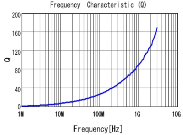
■ LQW15AN2N2B80 Q
