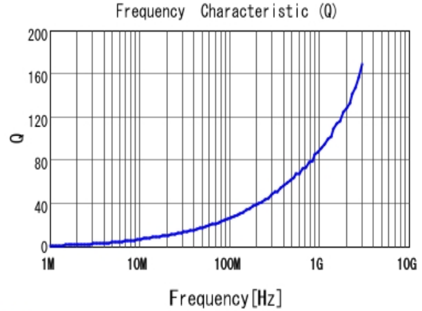
■ LQW15AN2N2C80 Q
