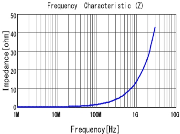
■ LQW15AN2N2C80 |Z|
