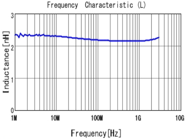
■ LQW15AN2N2C80 L
