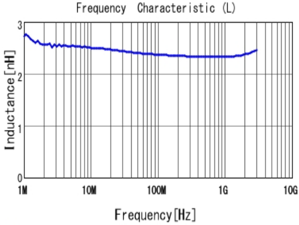
■ LQW15AN2N4C80 L
