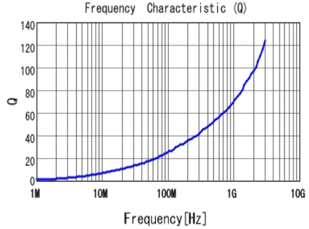
■ LQW15AN2N4C80 Q
