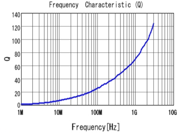
■ LQW15AN2N4G80 Q
