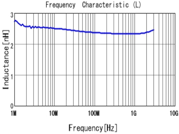
■ LQW15AN2N4G80 L
