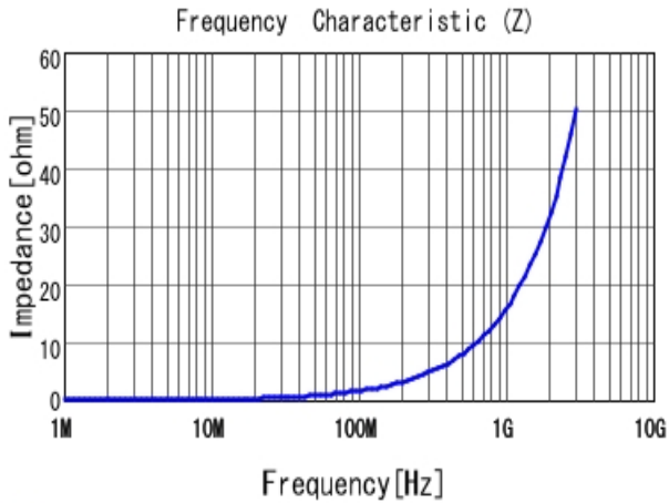
■ LQW15AN2N6C80 |Z|
