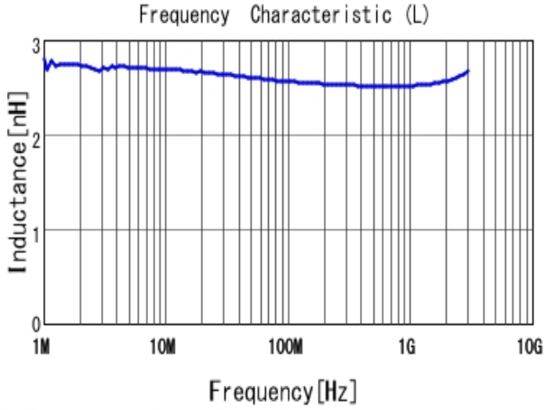
■ LQW15AN2N6C80 L
