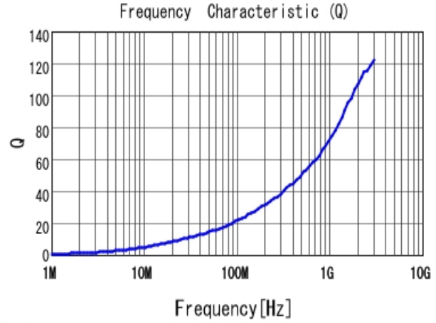
■ LQW15AN2N6C80 Q
