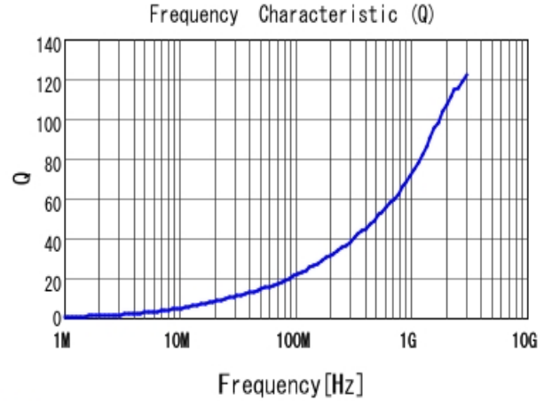
■ LQW15AN2N6G80 Q
