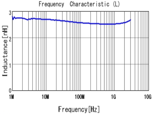
■ LQW15AN2N6G80 L
