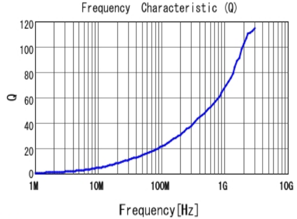
■ LQW15AN2N7B80 Q
