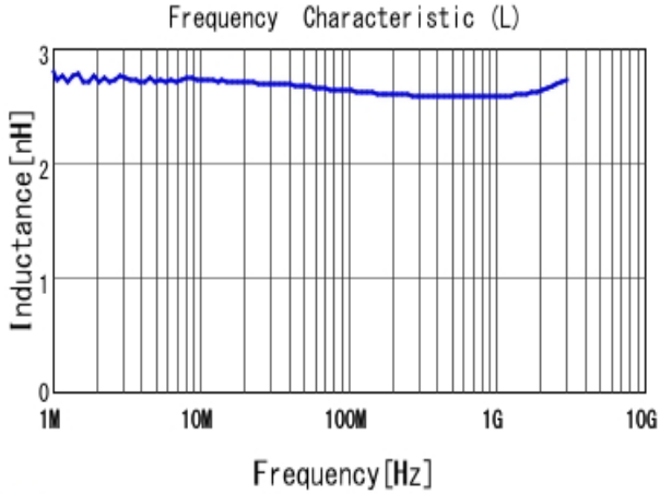
■ LQW15AN2N7B80 L
