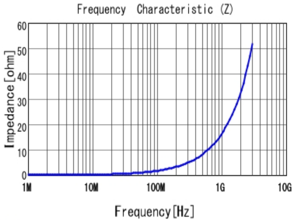
■ LQW15AN2N7D80 |Z|
