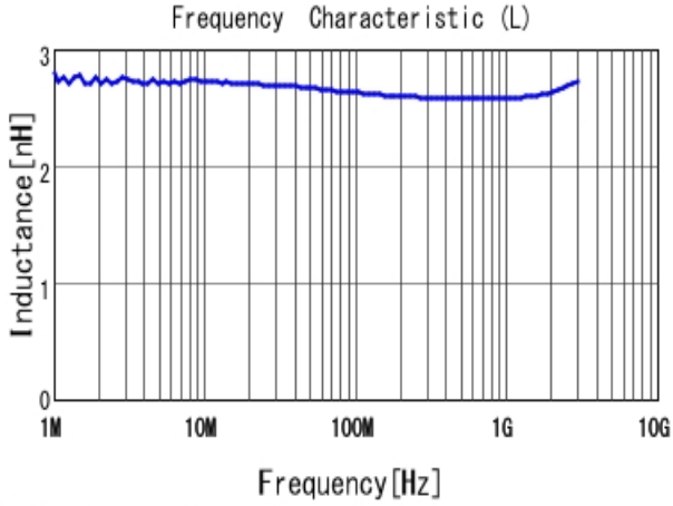
■ LQW15AN2N7D80 L
