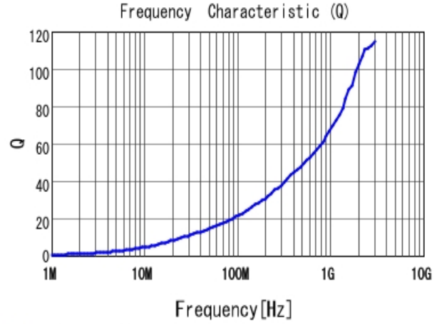
■ LQW15AN2N7D80 Q
