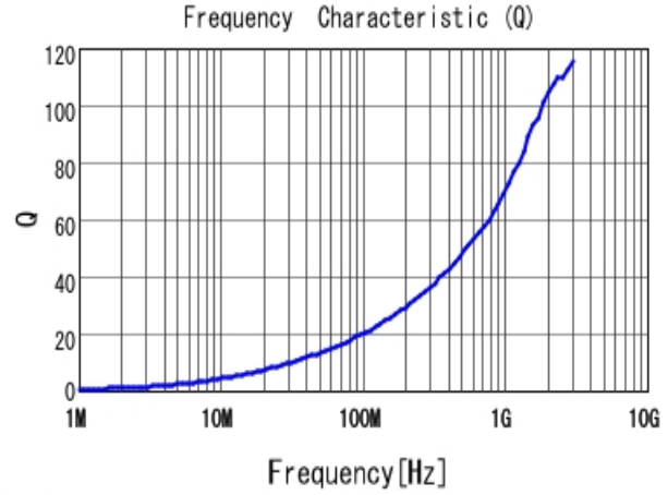
■ LQW15AN2N8B80 Q
