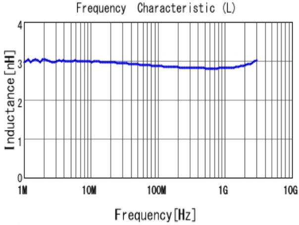
■ LQW15AN2N8B80 L
