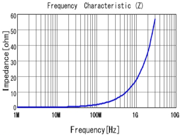
■ LQW15AN2N8B80 |Z|
