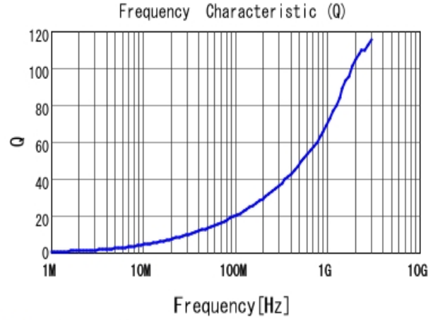
■ LQW15AN2N8D80 Q
