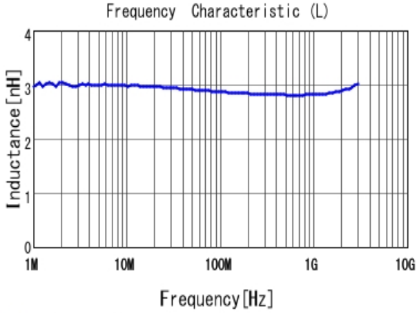
■ LQW15AN2N8D80 L
