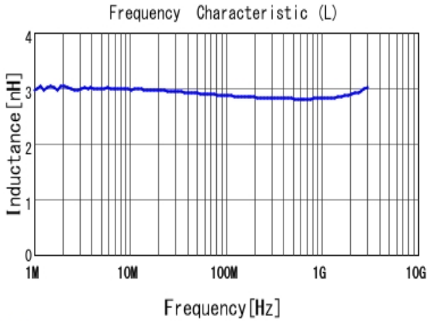
■ LQW15AN2N8G80 L
