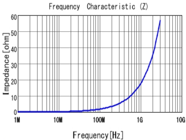
■ LQW15AN2N8G80 |Z|
