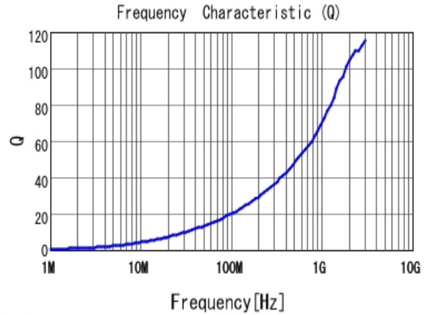
■ LQW15AN2N8G80 Q
