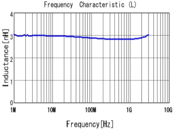
■ LQW15AN2N9B80 L
