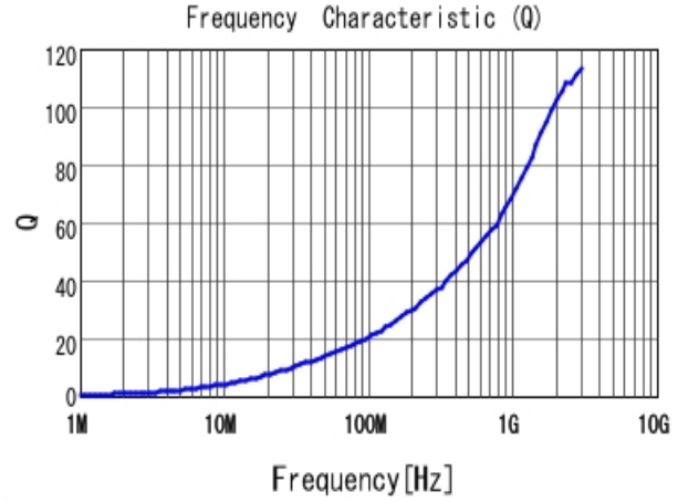
■ LQW15AN2N9B80 Q
