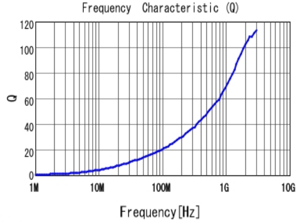
■ LQW15AN2N9C80 Q
