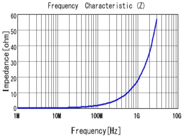
■ LQW15AN2N9C80 |Z|
