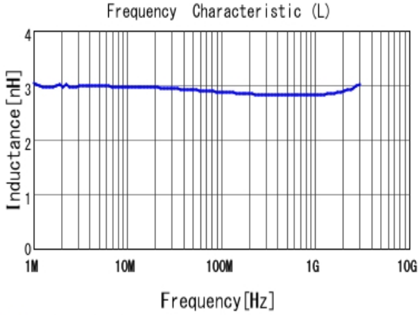
■ LQW15AN2N9C80 L
