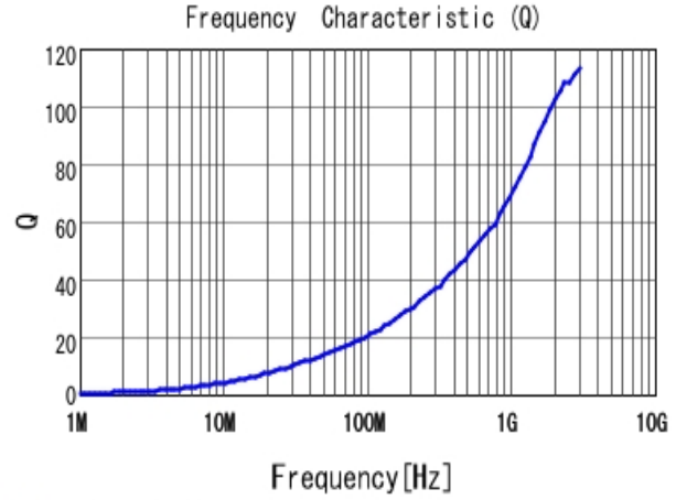
■ LQW15AN2N9D80 Q
