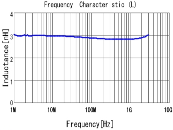
■ LQW15AN2N9D80 L
