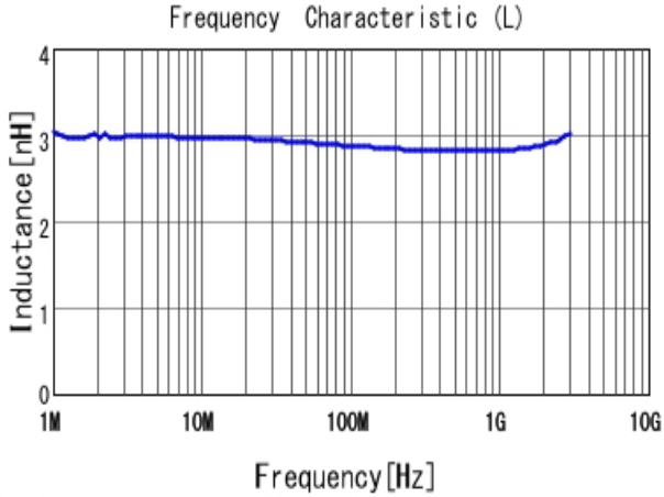
■ LQW15AN2N9G80 L
