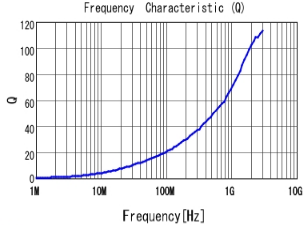
■ LQW15AN2N9G80 Q
