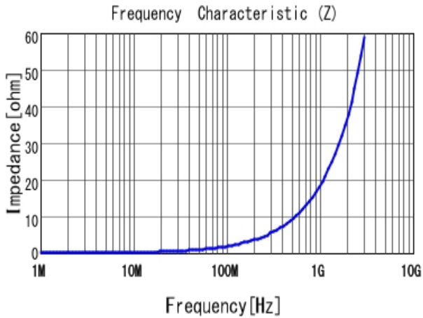
■ LQW15AN3N0C80 |Z|
