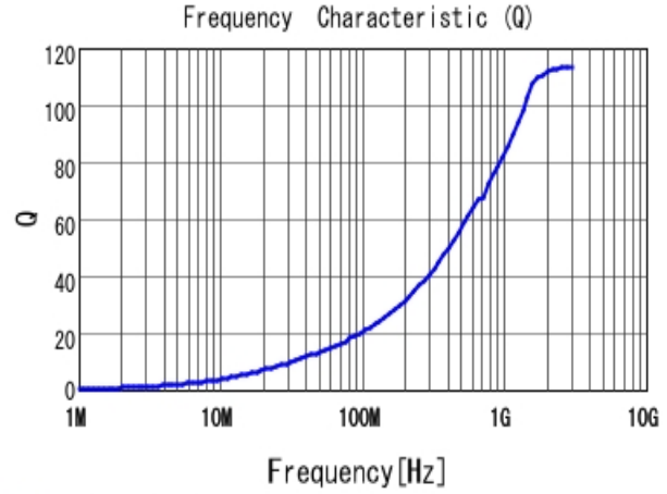
■ LQW15AN3N0C80 Q
