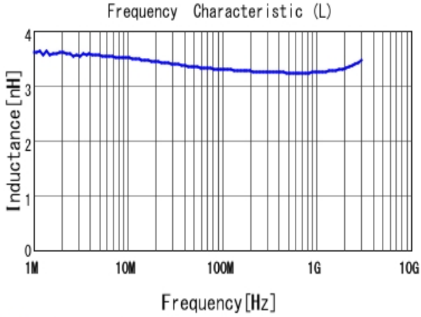
■ LQW15AN3N3B80 L
