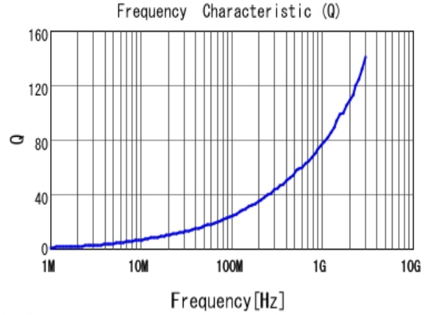
■ LQW15AN3N3B80 Q
