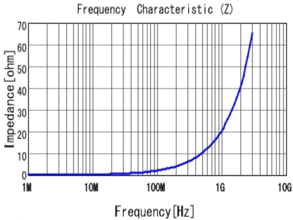
■ LQW15AN3N3B80 |Z|
