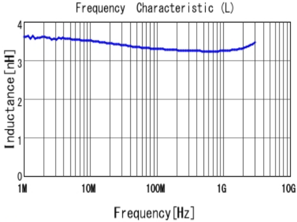
■ LQW15AN3N3C80 L
