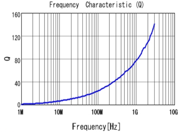
■ LQW15AN3N3C80 Q
