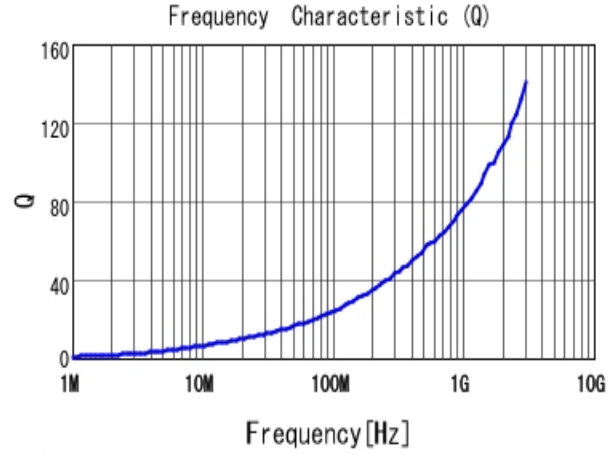
■ LQW15AN3N3D80 Q
