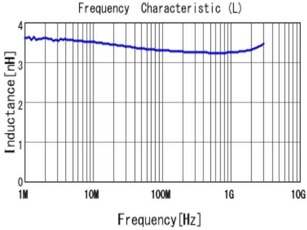
■ LQW15AN3N3D80 L
