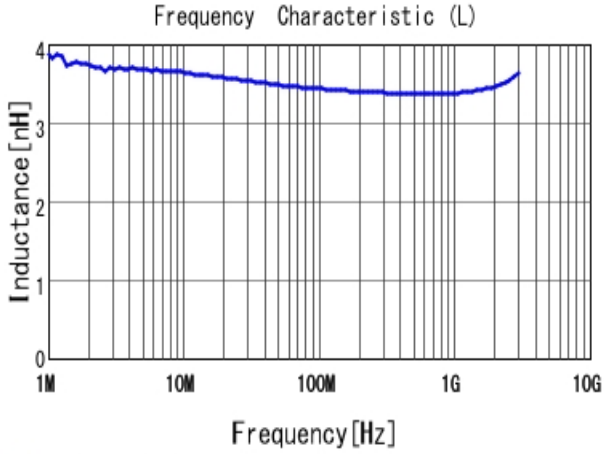
■ LQW15AN3N4C80 L
