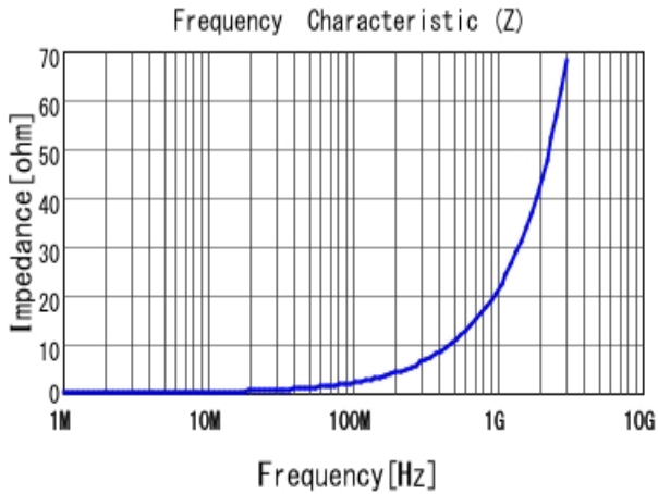
■ LQW15AN3N4C80 |Z|
