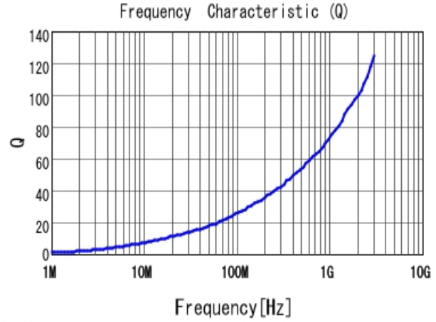
■ LQW15AN3N4C80 Q
