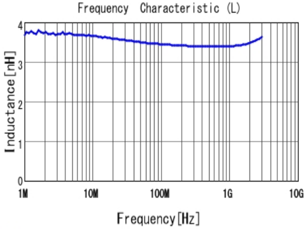
■ LQW15AN3N5B80 L
