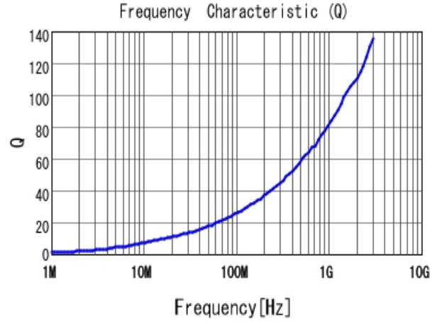
■ LQW15AN3N5B80 Q
