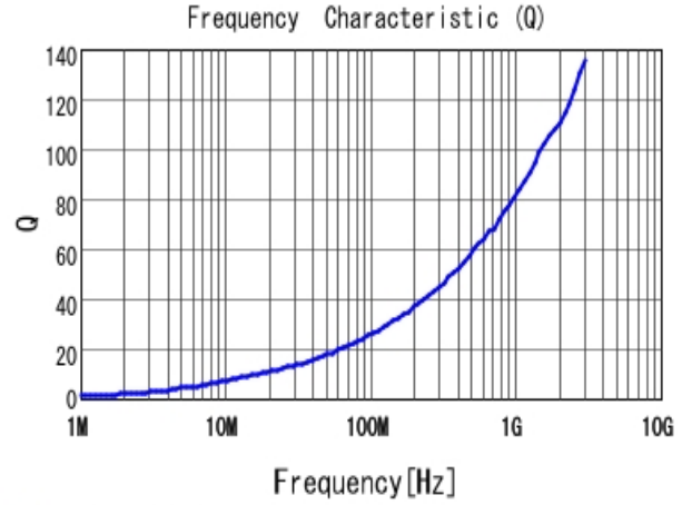
■ LQW15AN3N5C80 Q
