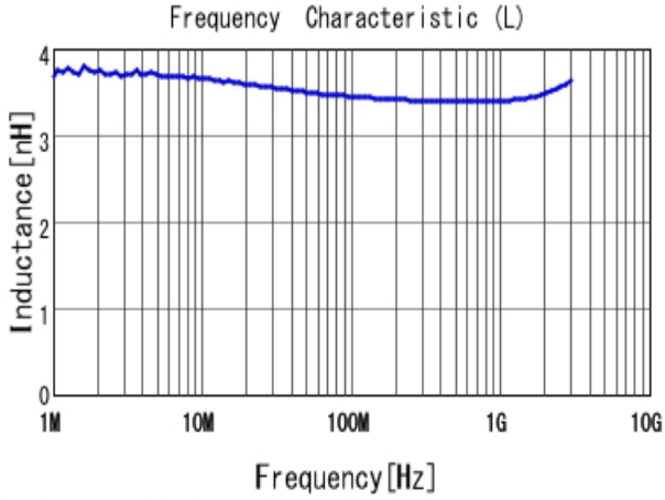
■ LQW15AN3N5C80 L
