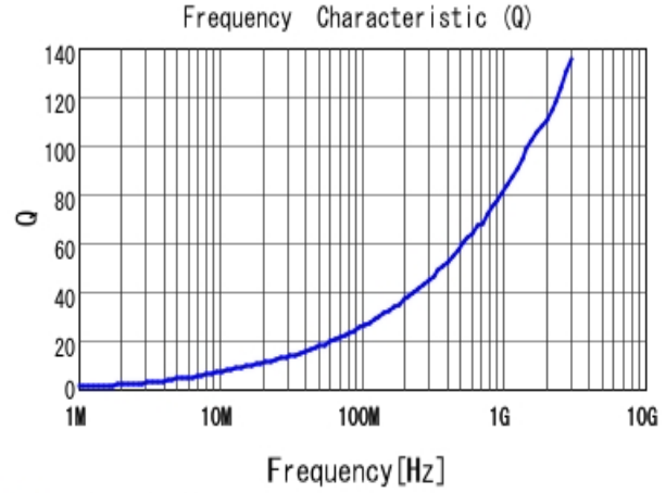
■ LQW15AN3N5D80 Q
