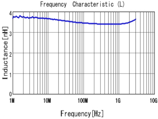
■ LQW15AN3N5D80 L
