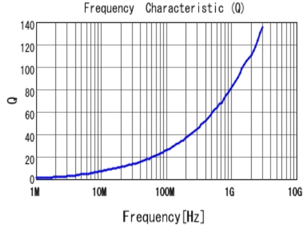
■ LQW15AN3N5G80 Q
