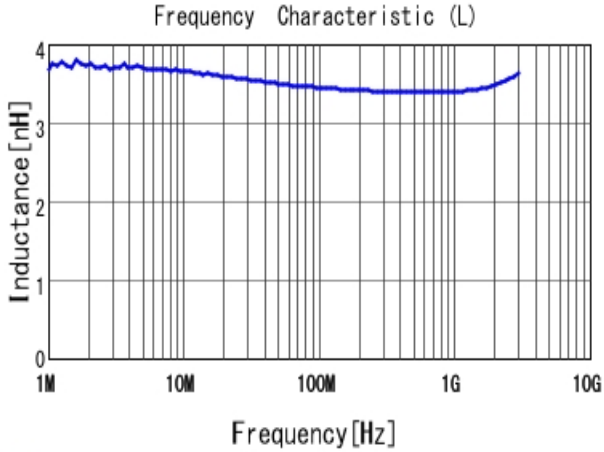
■ LQW15AN3N5G80 L
