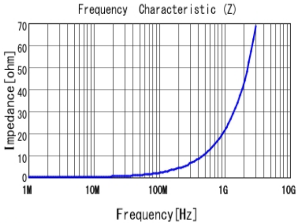
■ LQW15AN3N5G80 |Z|
