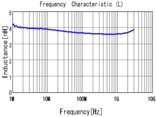
■ LQW15AN3N6B80 L
