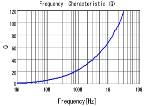
■ LQW15AN3N6B80 Q
