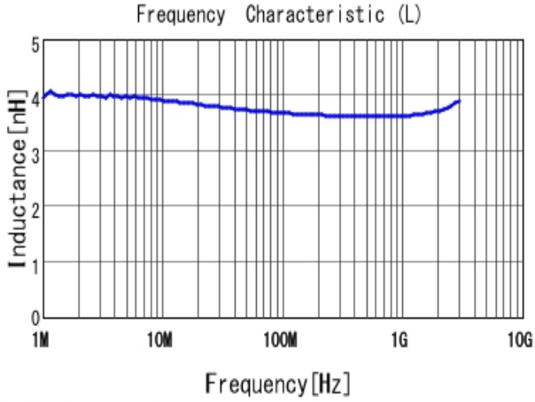
■ LQW15AN3N7C80 L
