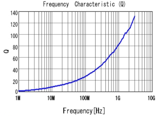
■ LQW15AN3N7C80 Q
