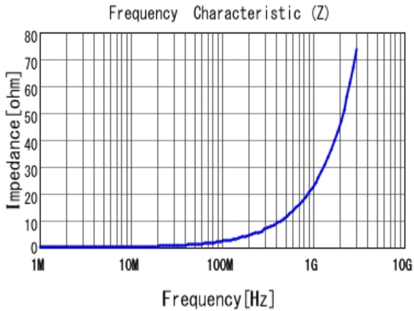
■ LQW15AN3N7C80 |Z|
