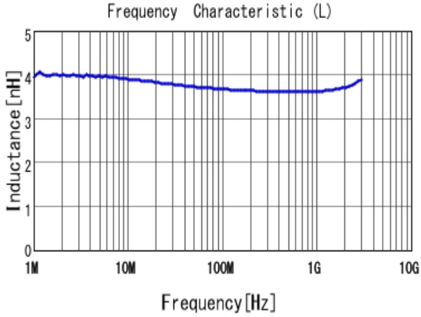
■ LQW15AN3N7D80 L
