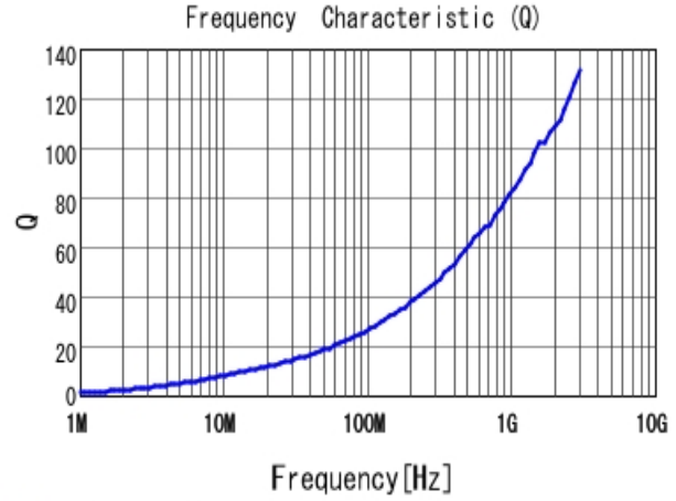
■ LQW15AN3N7D80 Q
