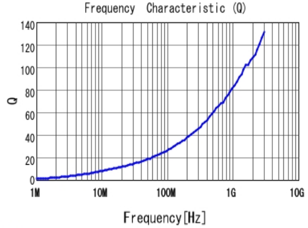
■ LQW15AN3N7G80 Q
