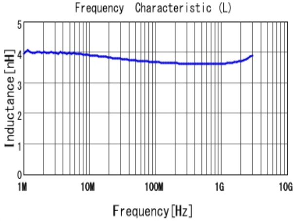
■ LQW15AN3N7G80 L
