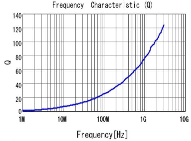
■ LQW15AN3N8C80 Q
