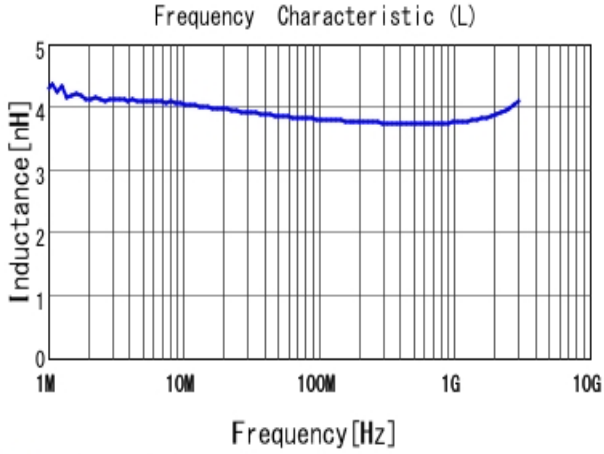
■ LQW15AN3N8C80 L
