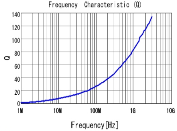
■ LQW15AN3N9B80 Q
