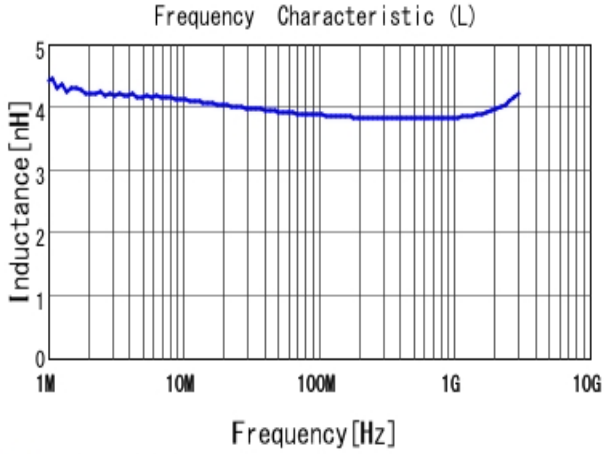
■ LQW15AN3N9B80 L
