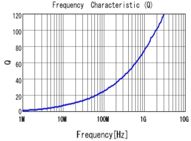
■ LQW15AN4N0B80 Q
