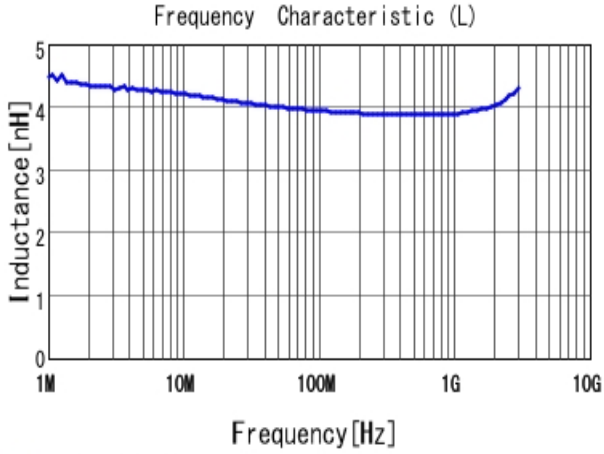
■ LQW15AN4N0D80 L
