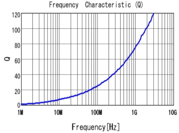
■ LQW15AN4N0D80 Q
