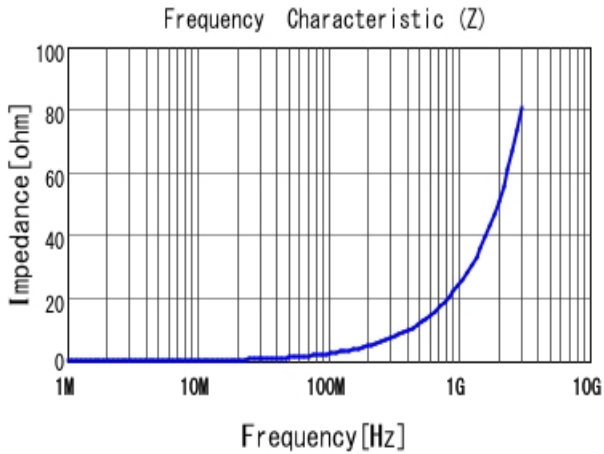
■ LQW15AN4N0G80 |Z|
