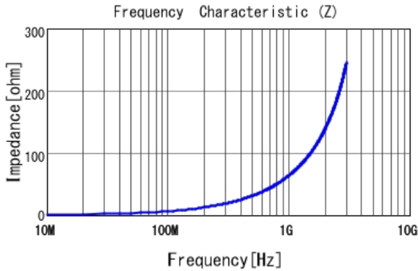
LQW18AN10NG00 |Z|
