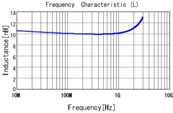
LQW18AN10NG00 L
