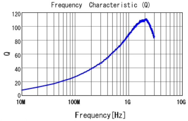
LQW18AN10NG00 Q
