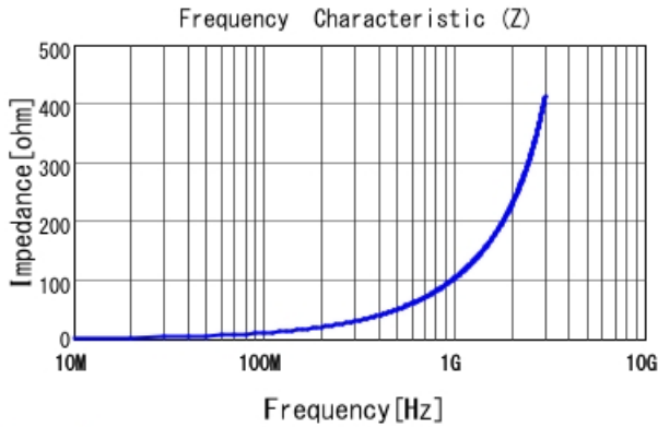
LQW18AN16NJ00 |Z|
