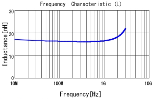
LQW18AN16NJ00 L
