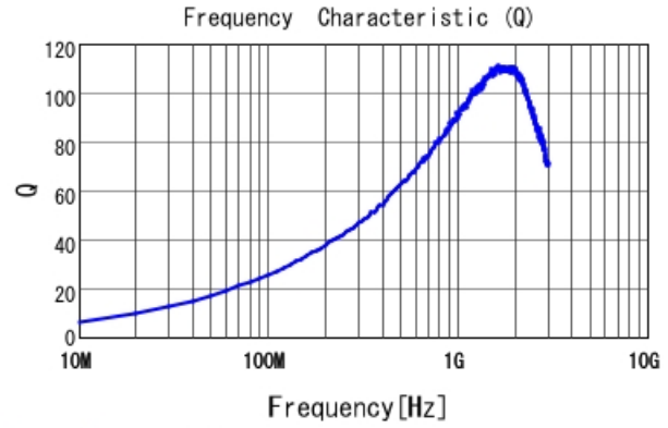
LQW18AN16NJ00 Q
