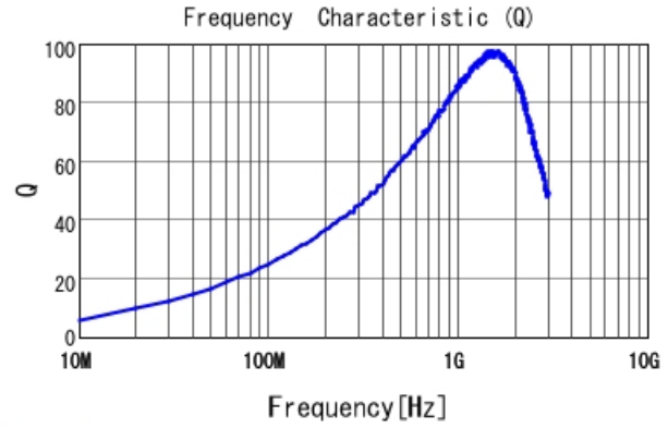
LQW18AN18NJ00 Q
