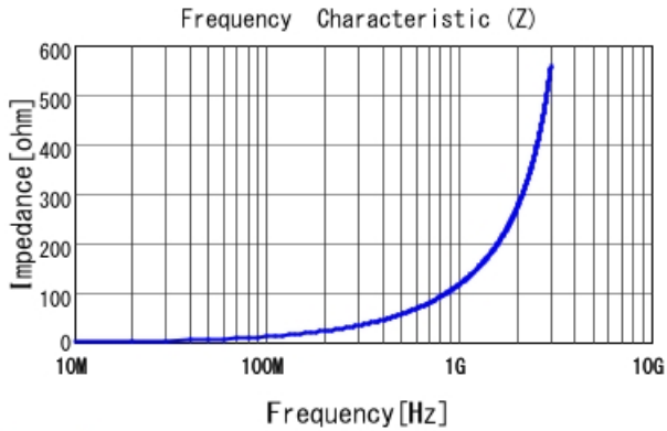
LQW18AN18NJ00 |Z|
