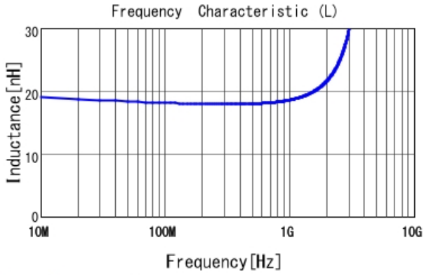
LQW18AN18NJ00 L
