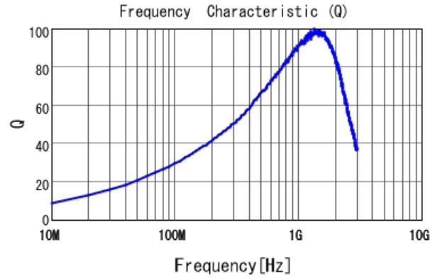
LQW18AN20NG00 Q
