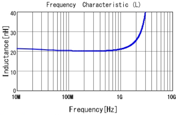
LQW18AN20NG00 L
