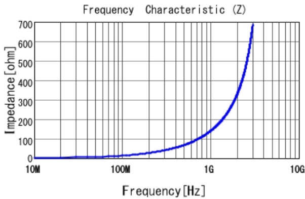
LQW18AN22NG00 |Z|
