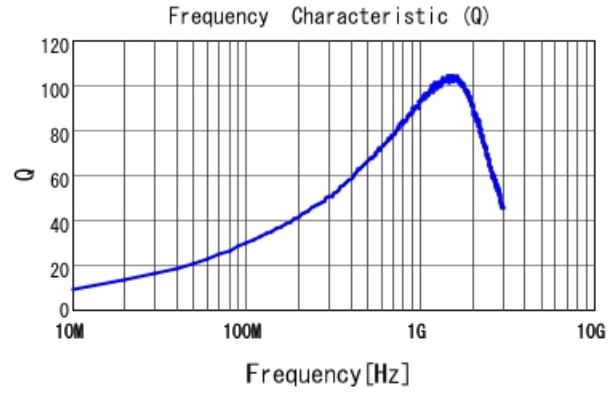
LQW18AN22NG00 Q
