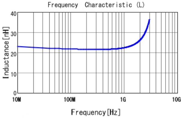
LQW18AN22NG00 L
