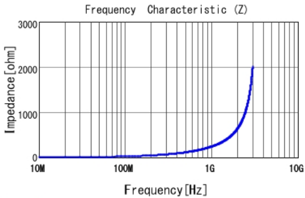
LQW18AN36NJ00 |Z|
