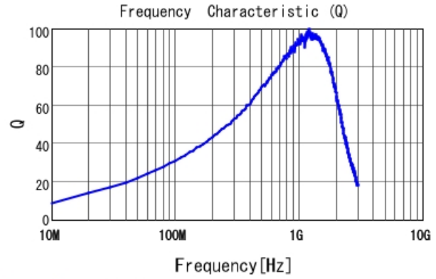
LQW18AN36NJ00 Q
