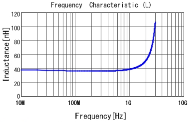
LQW18AN36NJ00 L
