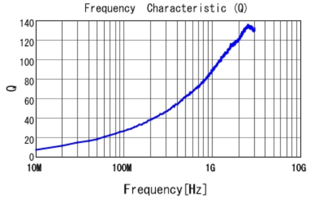
LQW18AN4N3C00 Q
