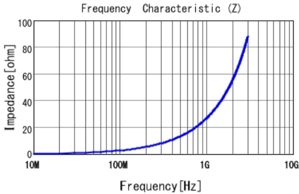
LQW18AN4N3C00 |Z|
