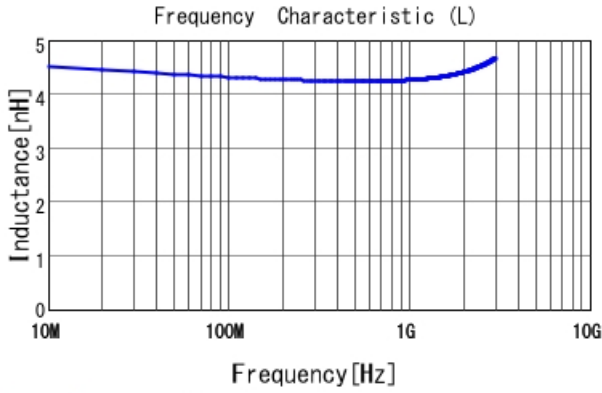
LQW18AN4N3C00 L
