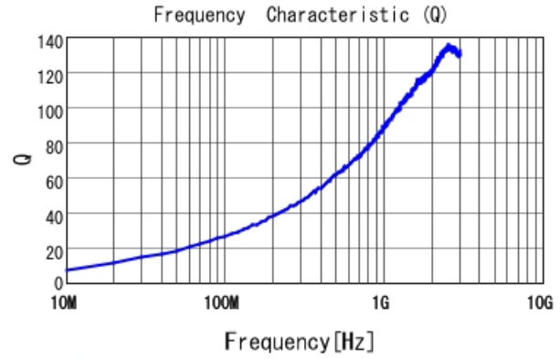
LQW18AN4N3D00 Q
