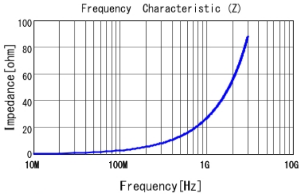
LQW18AN4N3D00 |Z|
