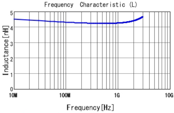
LQW18AN4N3D00 L
