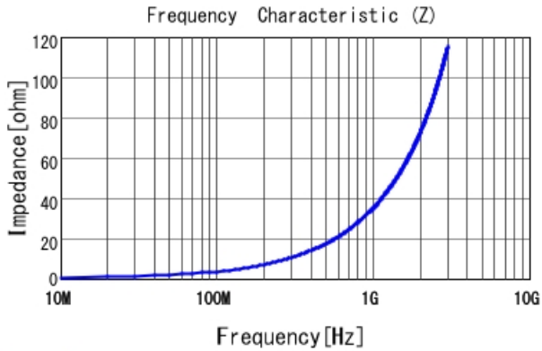
LQW18AN5N6D00 |Z|
