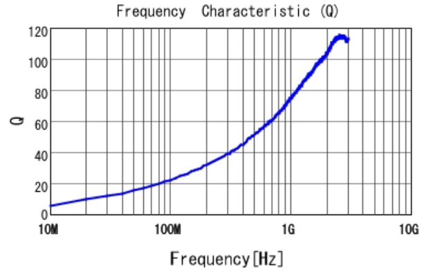
LQW18AN5N6D00 Q
