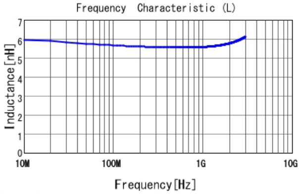
LQW18AN5N6D00 L
