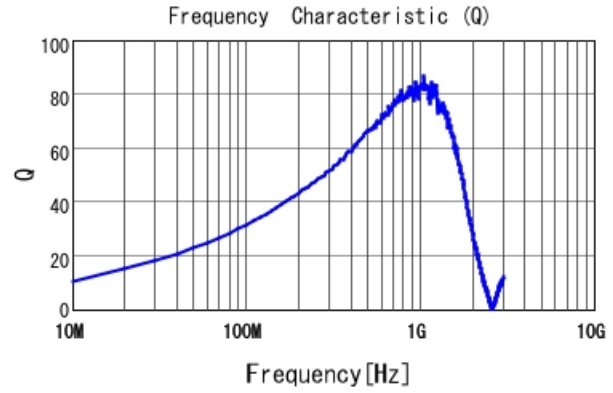
LQW18AN68NG00 Q
