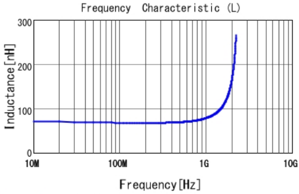
LQW18AN68NG00 L
