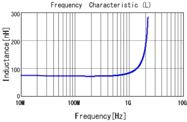
LQW18AN72NG00 L
