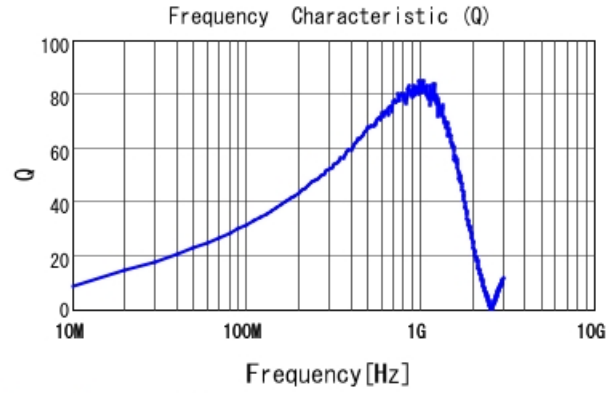
LQW18AN72NG00 Q
