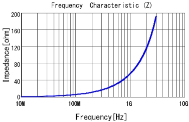
LQW18AN8N7C00 |Z|
