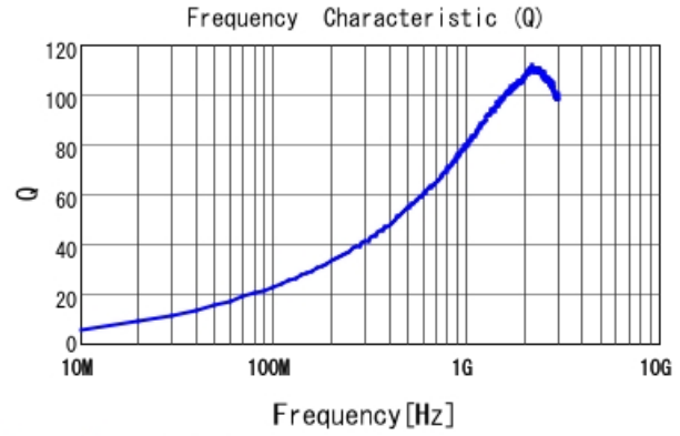
LQW18AN8N7C00 Q
