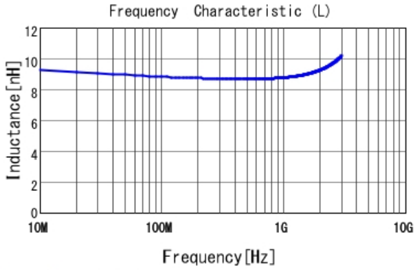
LQW18AN8N7C00 L
